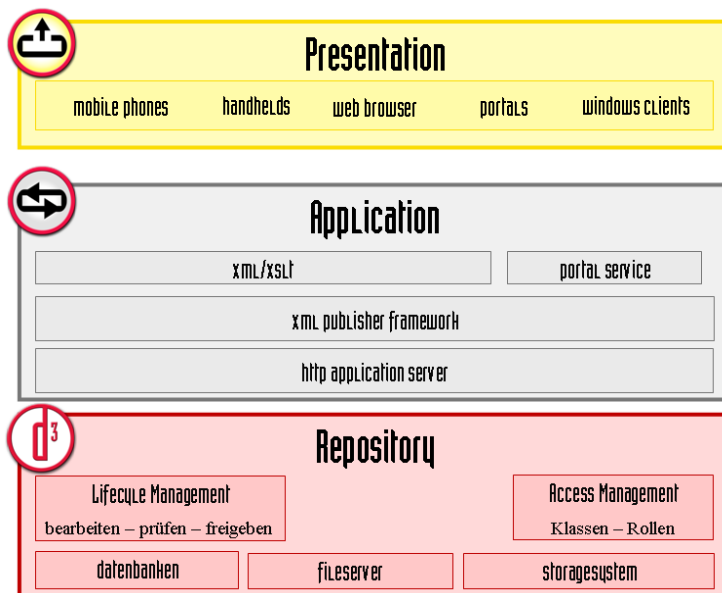
Abb. 2: d.3 web baut auf einem modernen XML-Framework und einem Applikationsserver auf.
